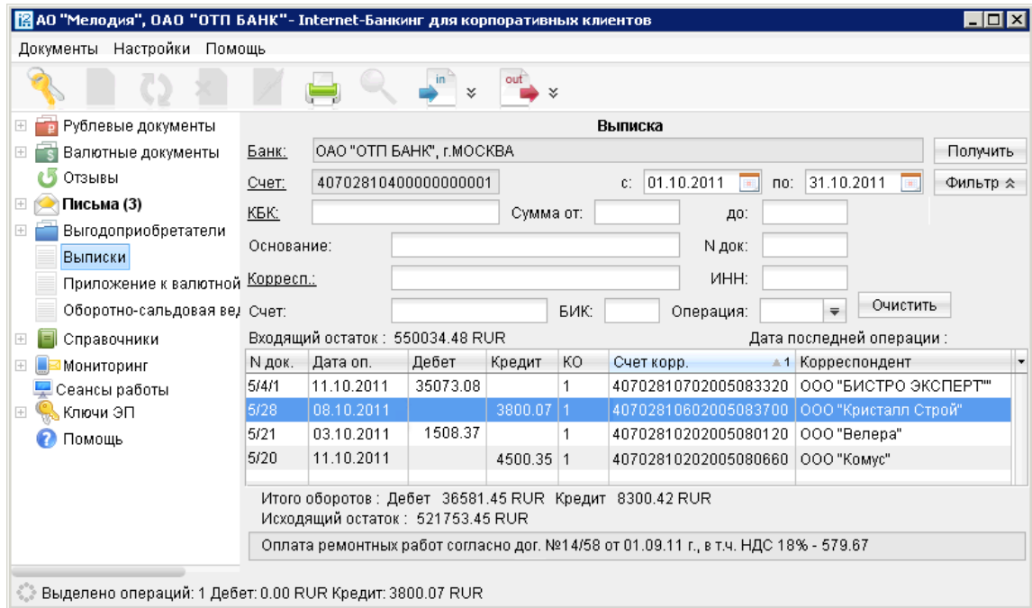
Рис. 18. Раздел "Выписки"
