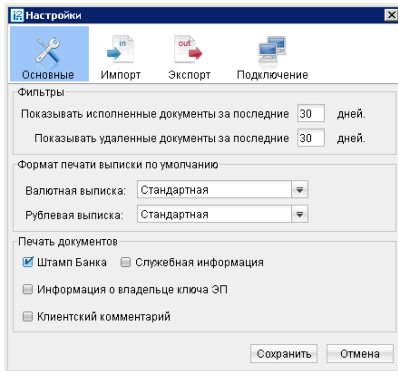
Рис. 14. Окно "Настройки"
